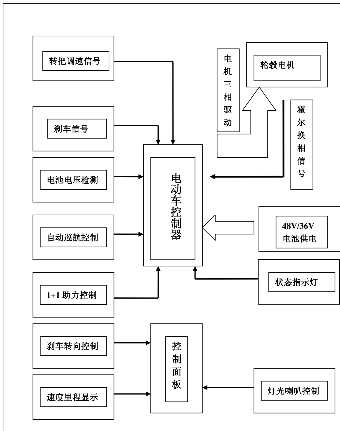
上海海尔集成电路电动车系统方案控制功能框图
